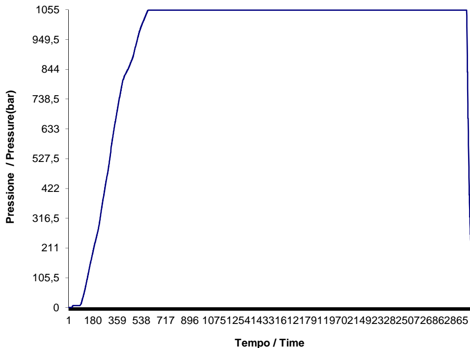
Andamento Pressione / Pressure Trend
